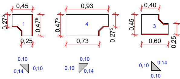
DETALHE 1- Cantos (chanfro 14cm)
