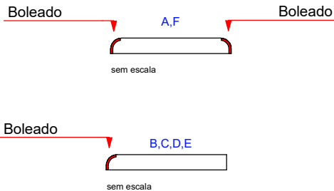
DETALHE 3- Acabamento
