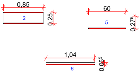
DETALHE 2- medida peça padrão
