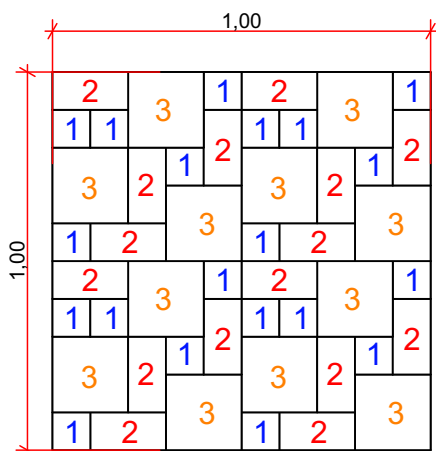
PAGINAÇÃO - 1,00m²
