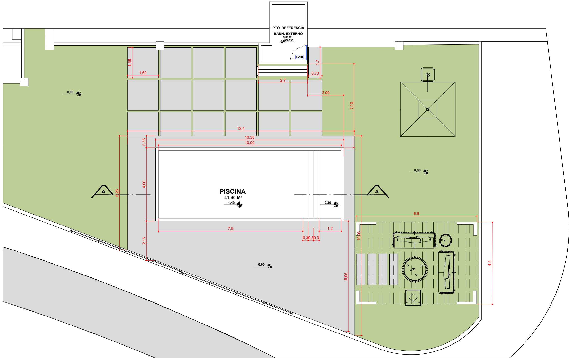
PLANTA TÉRREO - ESPECIFICAÇÃO PISCINA ESC 1:100
