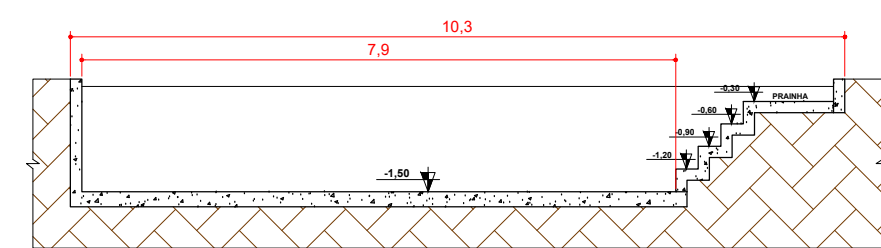
CORTE AA ESC 1:100
