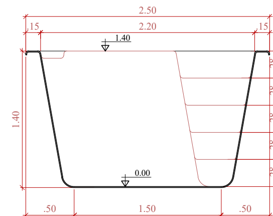
CORTE TRANSVERSAL
