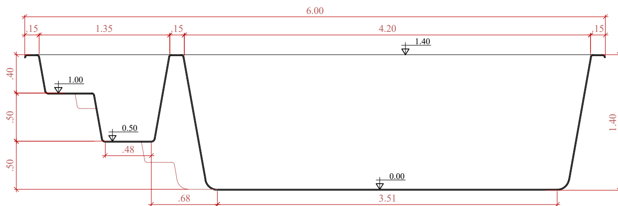
CORTE LONGITUDINAL
