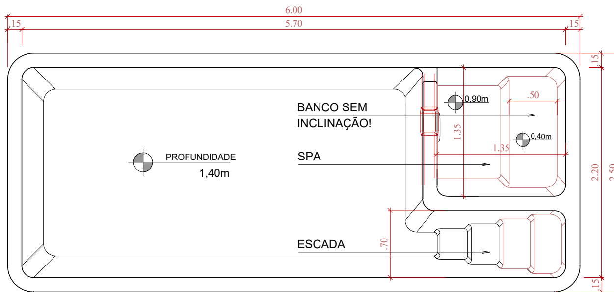
PLANTA - PISCINA LINHA TRADICIONAL COM SPA
