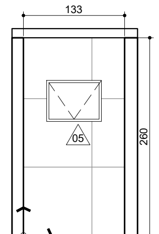
VISTA 15 - BAN. SUÍTE 01 ESC: 1/50
