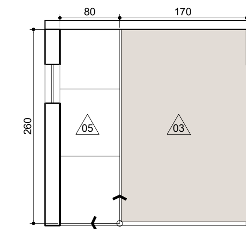
VISTA 09 - LAVABO EXTERNO ESC: 1/50
