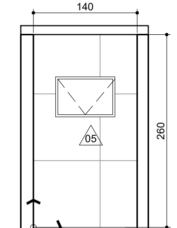
VISTA 20 - BAN. SUÍTE 03 ESC: 1/50
