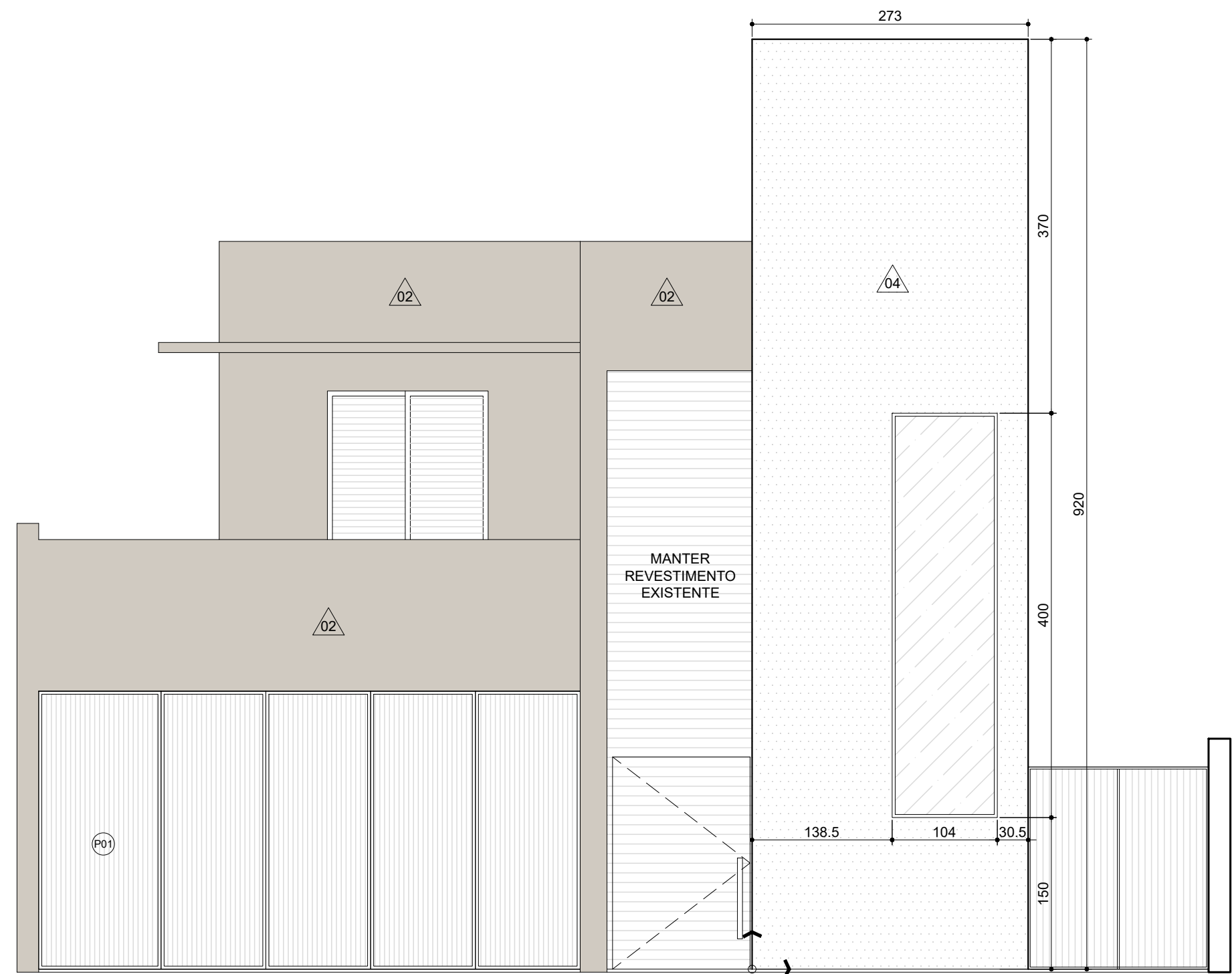
VISTA 01 - FACHADA FRONTAL ESC: 1/50
