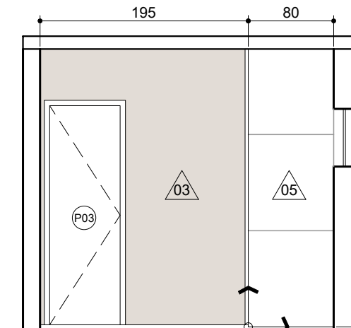
VISTA 14 - BANHO SUÍTE 01 ESC: 1/50
