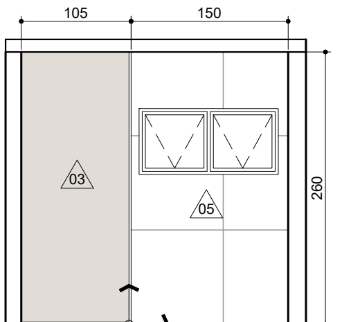
VISTA 18 - BAN. SUÍTE 02 ESC: 1/50
