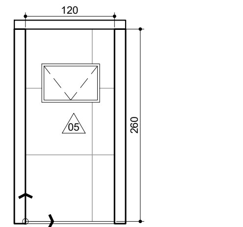
VISTA 08 - LAVABO EXTERNO ESC: 1/50
