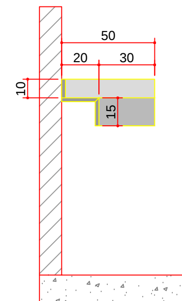
CORTE LAVATÓRIO
