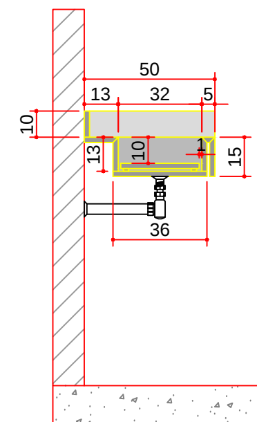
CORTE CUBA
