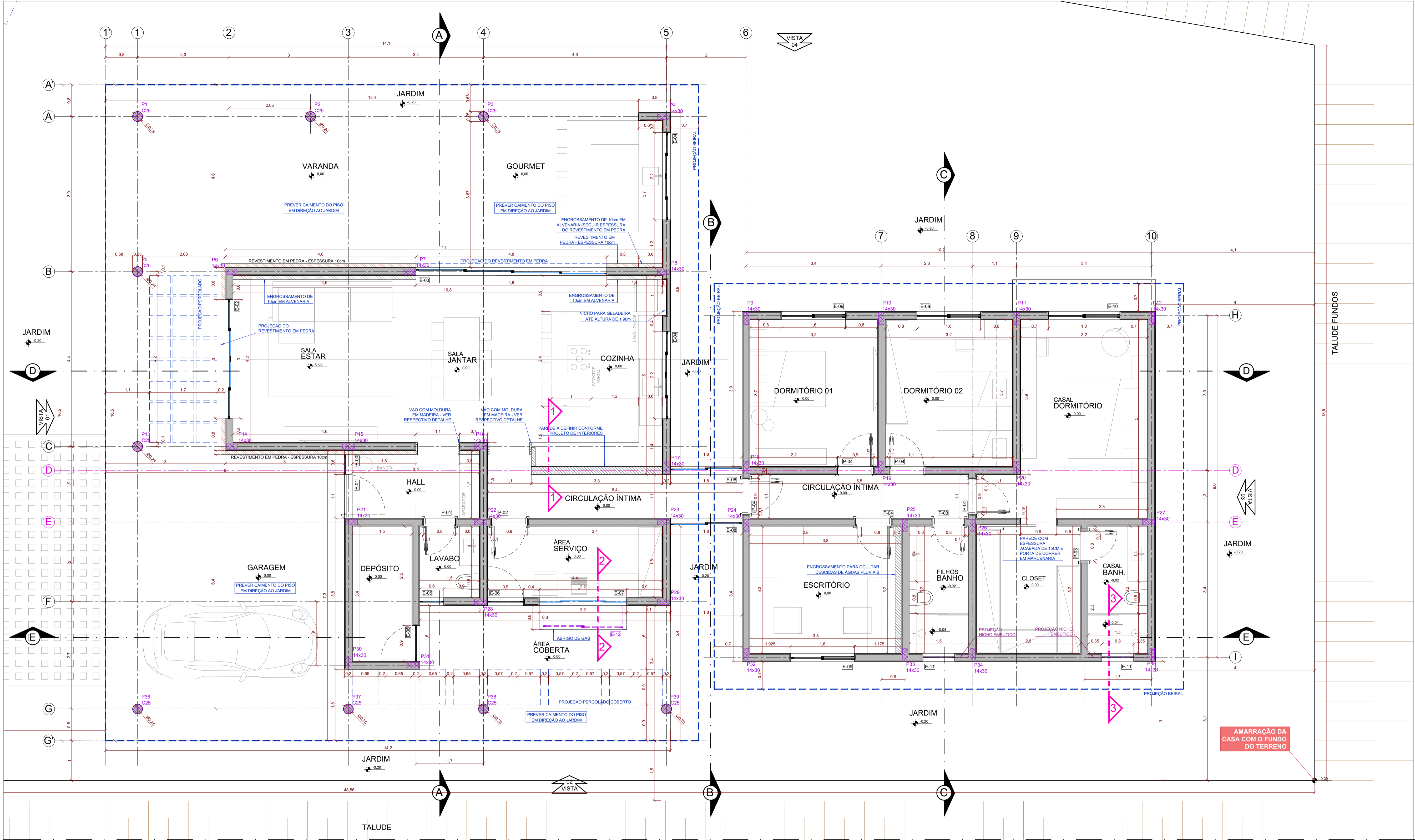
PLANTA TÉCNICA DE OBRA PAV. TÉRREO ESC 1:50
