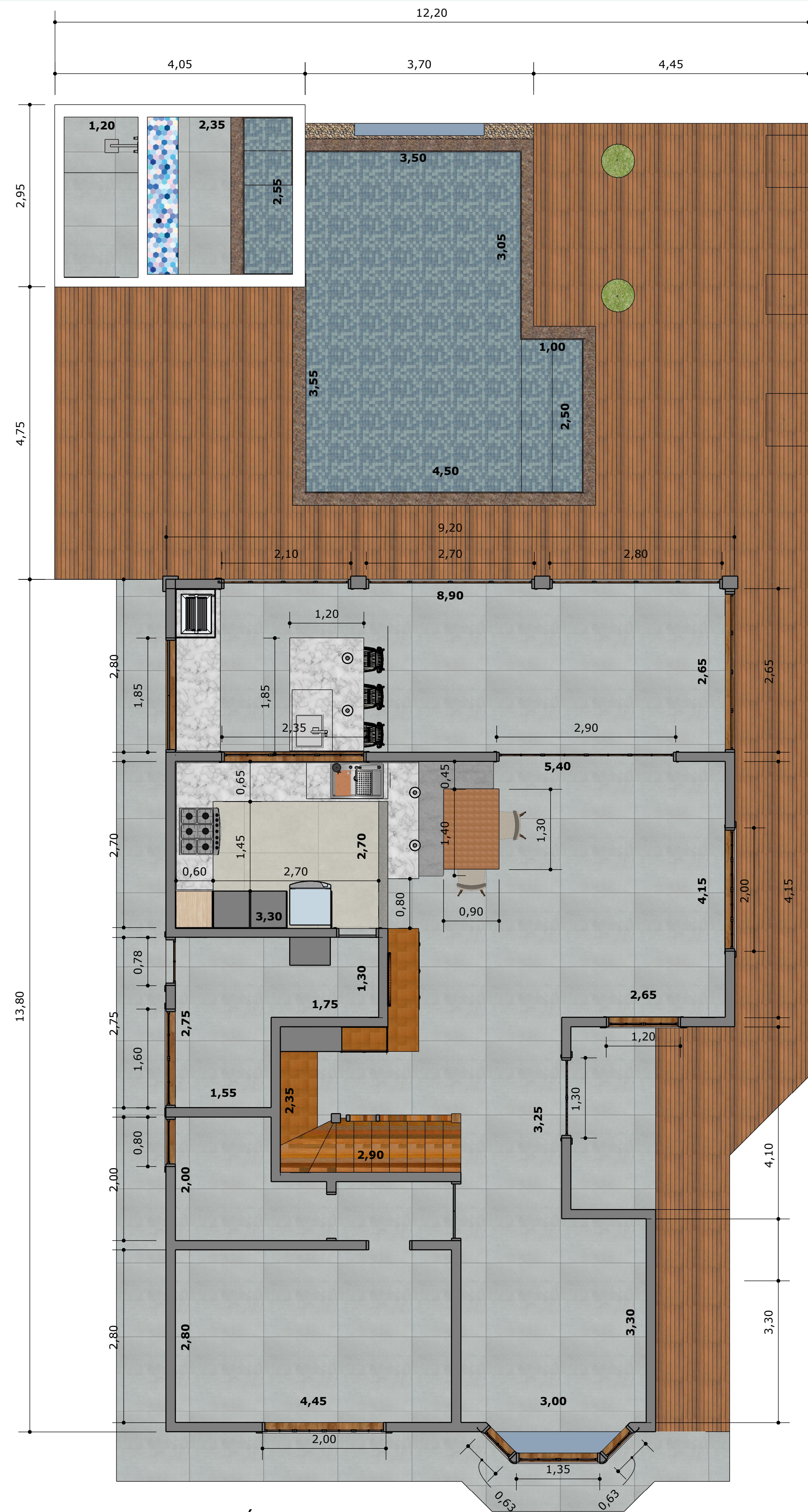
EP5 - PAV. TÉRREO PLANTA BAIXA Esc. 1:50
