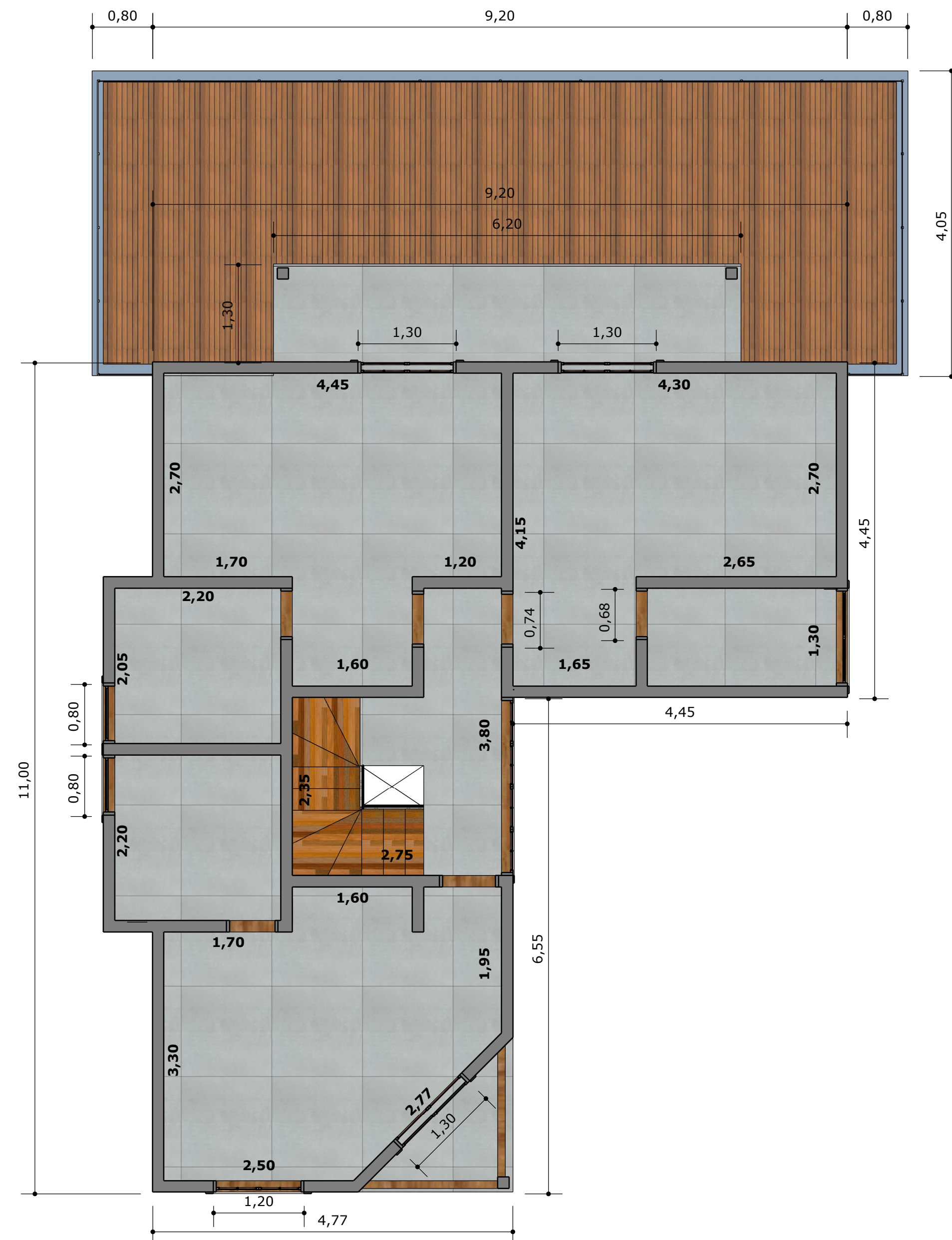
EP5 - PAV. SUPERIOR PLANTA BAIXA Esc. 1:50
