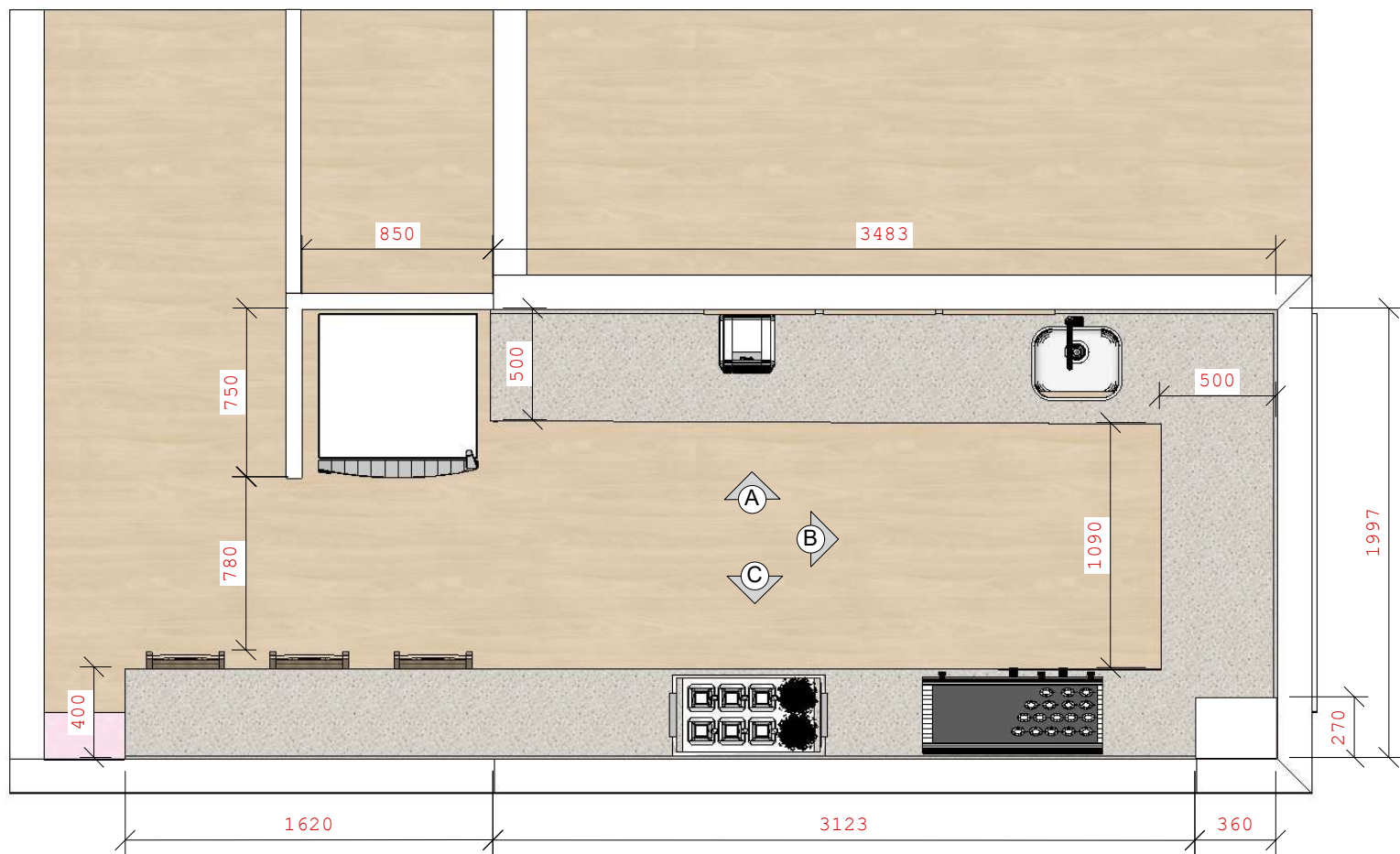
DETALHAMENTO PLANTA
