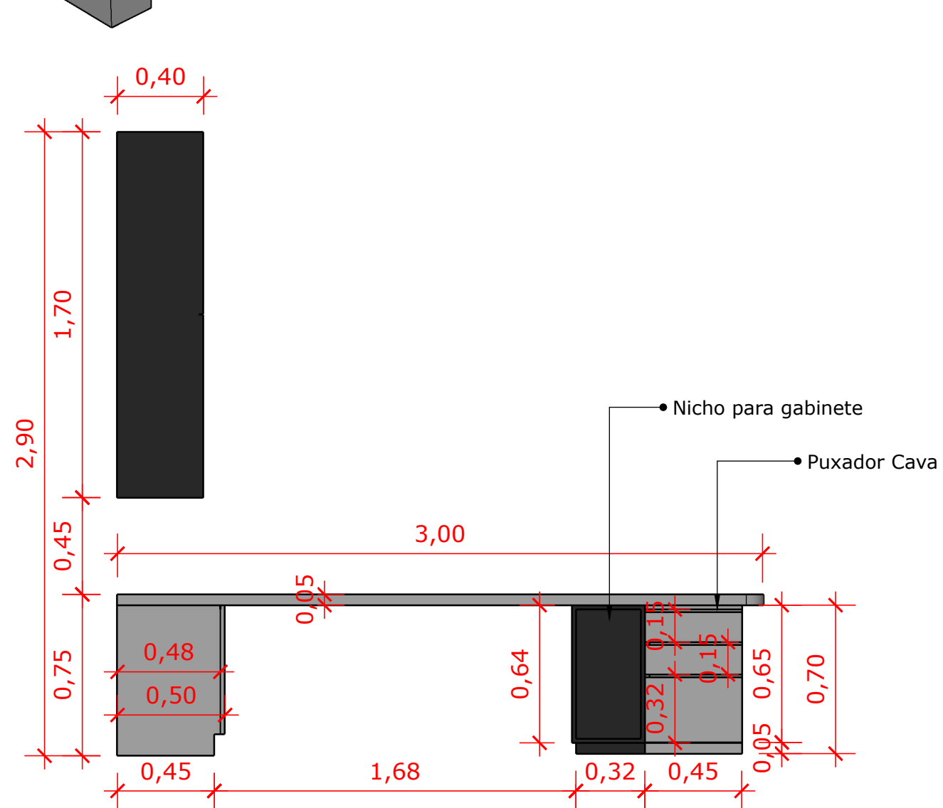
VISTA POSTERIOR
