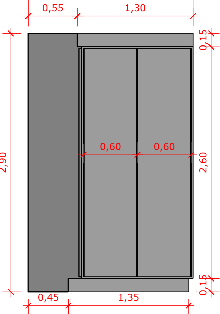
VISTA "B"
