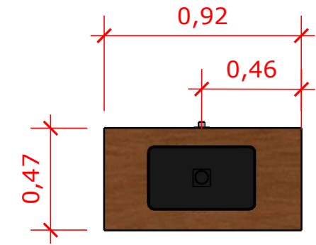
VISTA SUPERIOR
