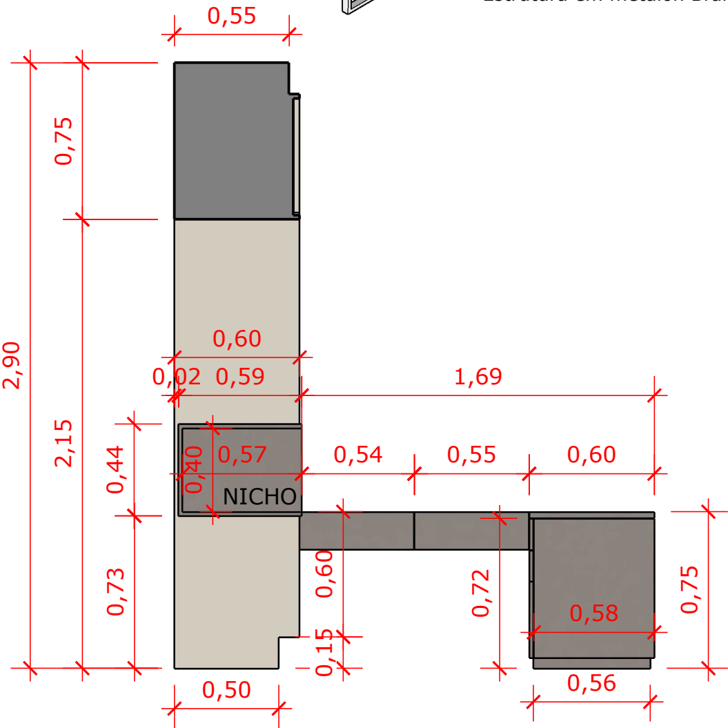
VISTA "A"
