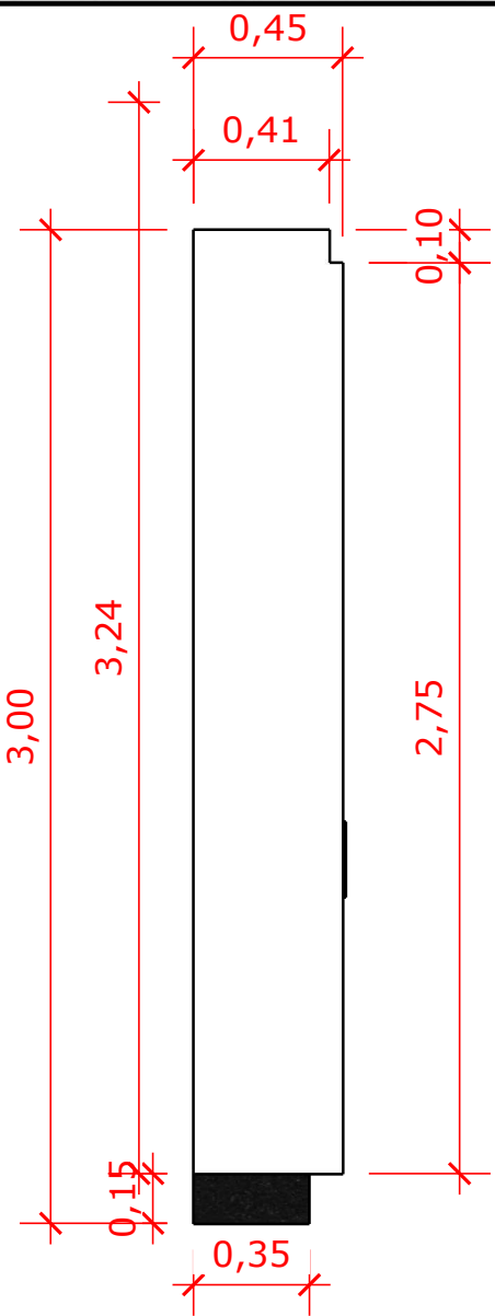
VISTAS LATERAIS
