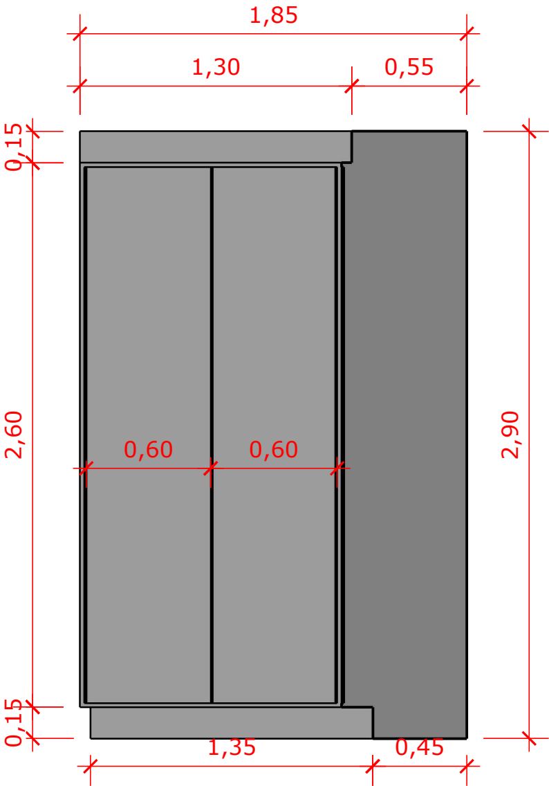
VISTA "A"
