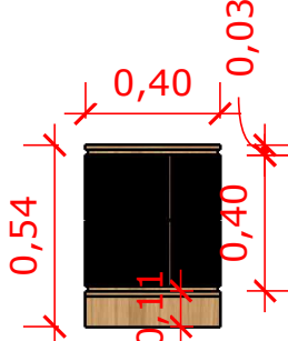
VISTAS LATERAIS
