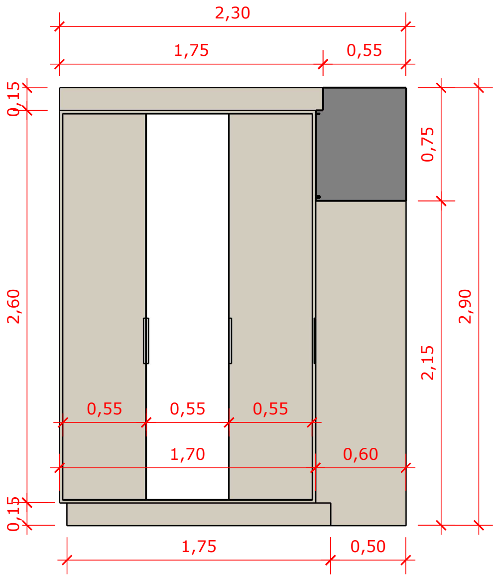
VISTA "B"
