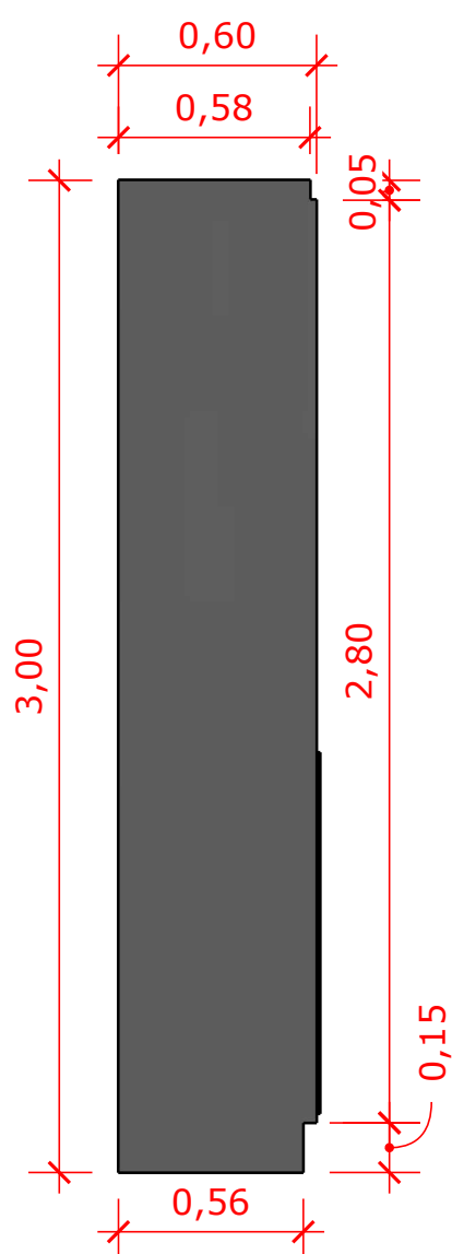
VISTAS LATERAIS
