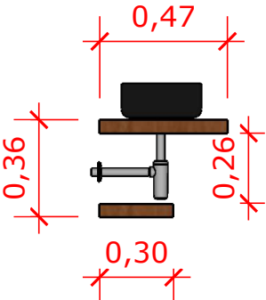
VISTAS LATERAIS
