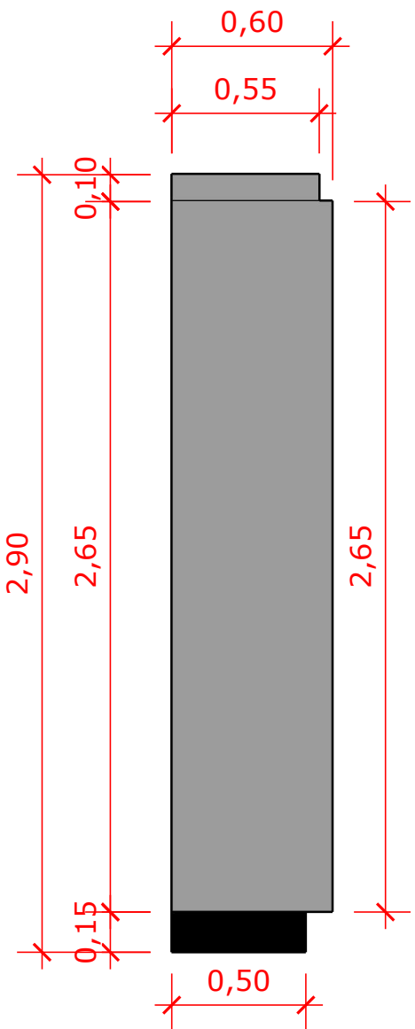
VISTAS LATERAIS
