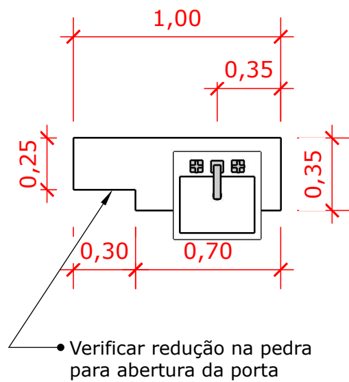
VISTA SUPERIOR
