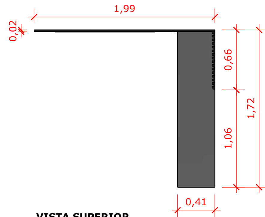
VISTA SUPERIOR
