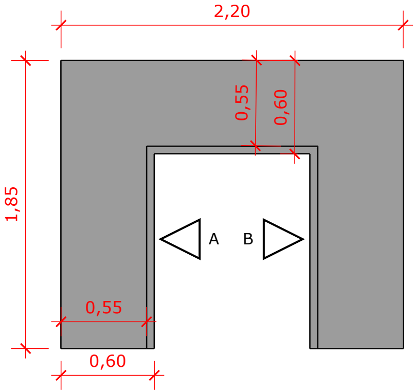
VISTA SUPERIOR
