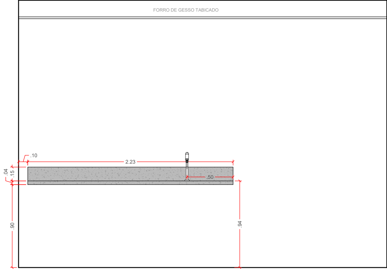
VISTA 02 - PEDRAS COZINHA E LAVANDERIA ESC: 1:25
