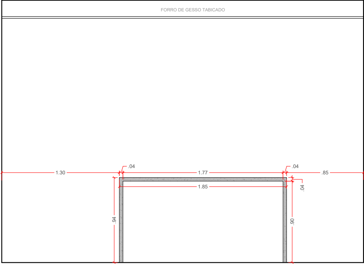
VISTA 03 - PEDRAS COZINHA E LAVANDERIA ESC: 1:25
